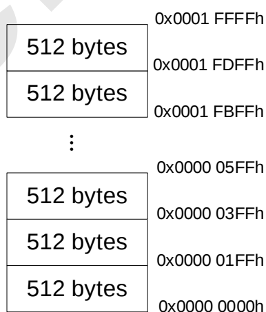
SC32F15G 系列 128 Kbytes APROM Sector 分区示意
